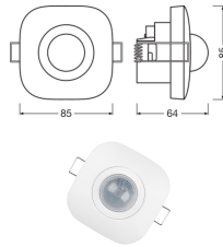
Tekniset tiedot Ledvance Vivares Zigbee Sensor | Presence
